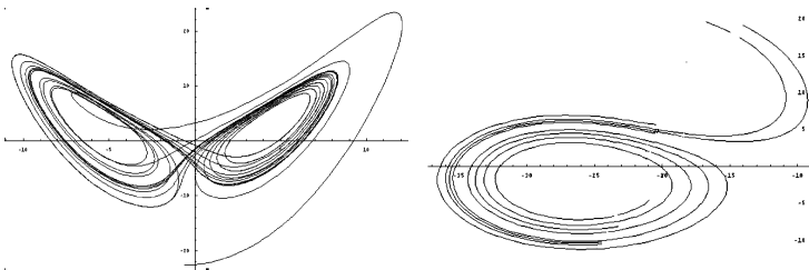
Рис. 2. Траектория системы с аттрактором Лоренца и подмножество ее сегментов
